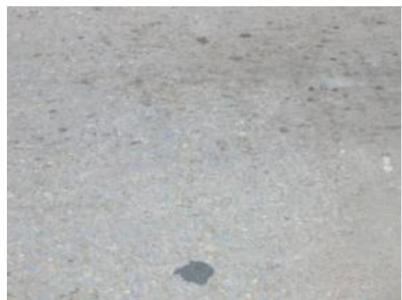
รูปที่ 4-79 ลักษณะการสึกกร่อนของผิวถนนจนเห็นเม็ดหินเกิดขึ้นทั่วสะพาน
