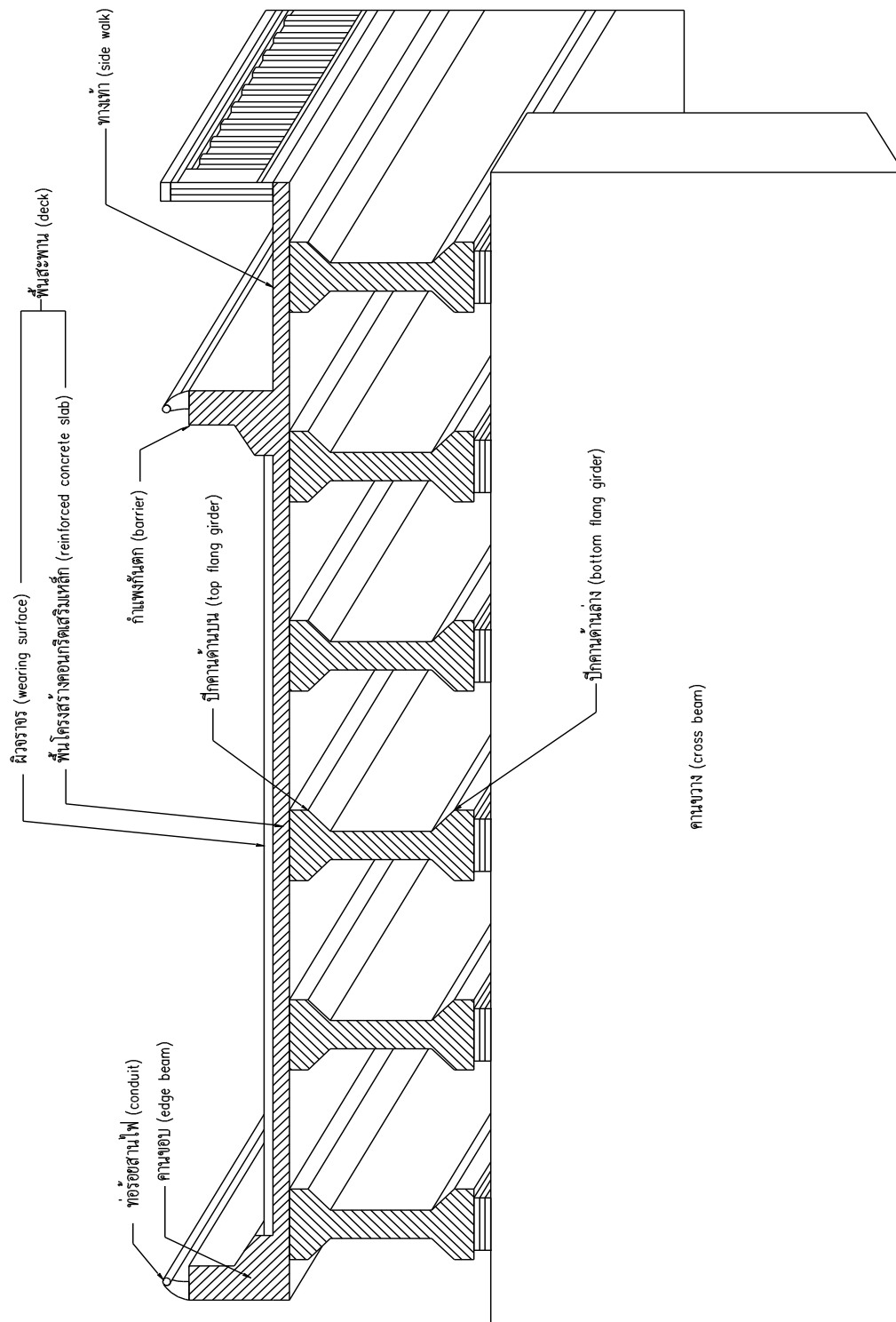
รูปที่ 2-40 องค์ประกอบโครงสร้างสะพานแบบคานคอกนกรัดอัดแรงรูปตัวไอ (I-Girder)
