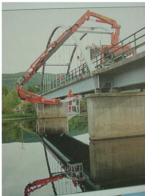
รูปที่ 3-15 แสดงการตรวจสอบโครงสร้างสะพานโดยการใช้รถกระเช้าพิเศษ
