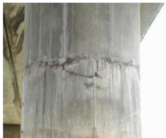
รูปที่ 4-47 การแตกร้าวช่วงกลางความยาวเสาตอม่อ
