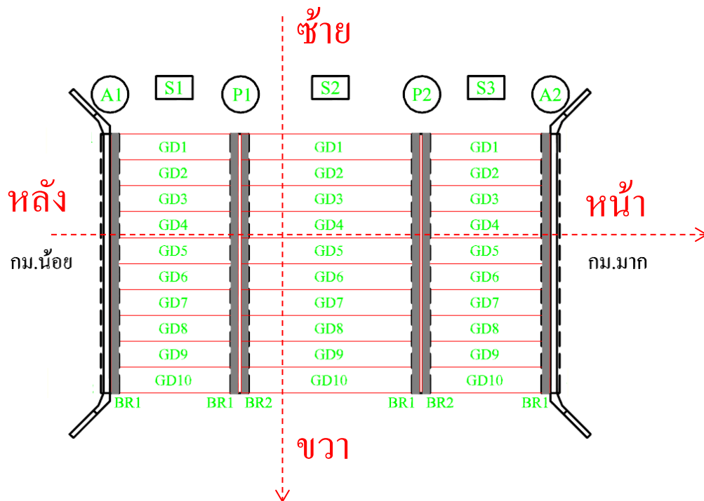
รูปที่ 3-22 ตัวอย่างการเรียงลำดับชิ้นส่วนจากช้ายไปขวาแล้วหลังไปหน้า
