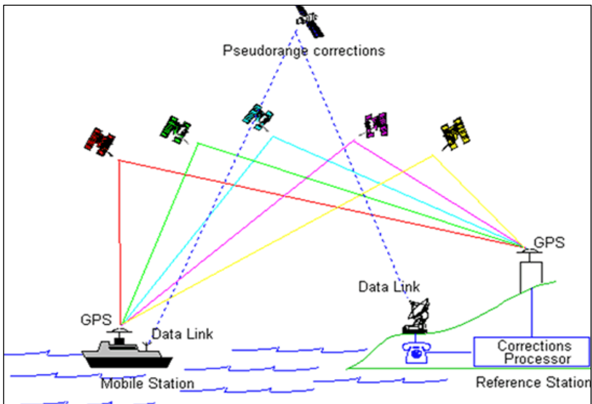
รูปที่ 2-30 หลักการทำงานของระบบรับพิกัดและค่าแก้ไข DGPS
