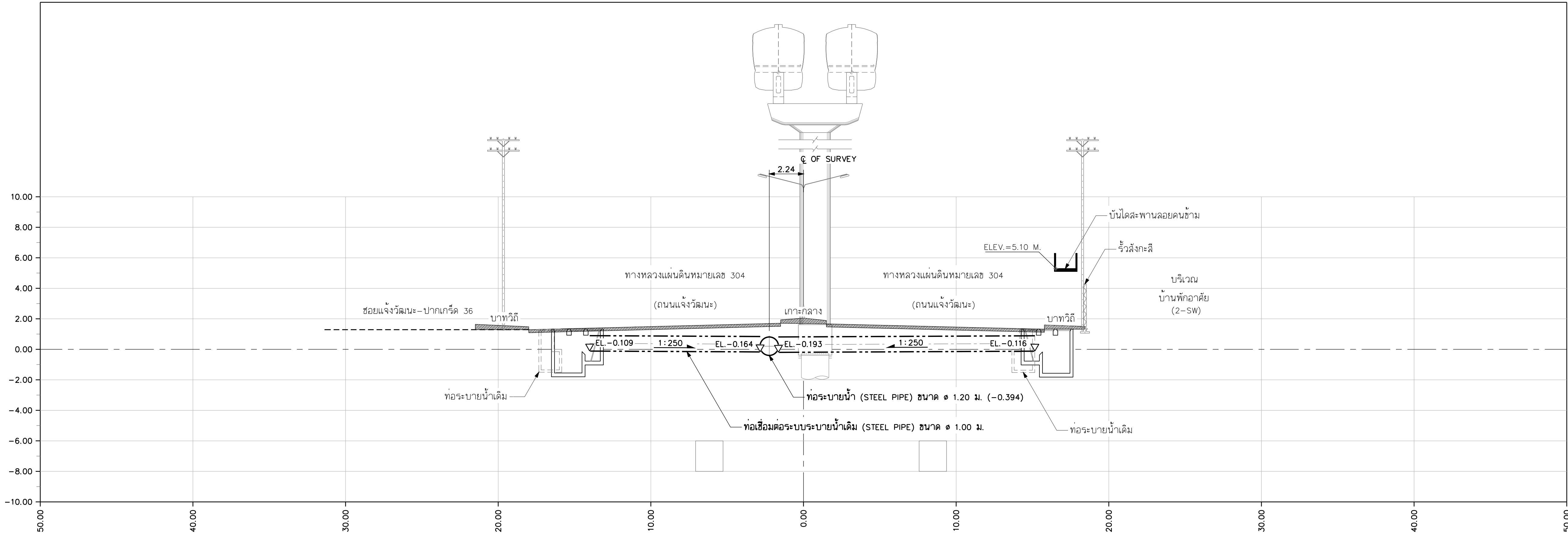
รูปตัดตามขวาง 9-9 กม. 6+043.270 มาตราส่วน 1:150
