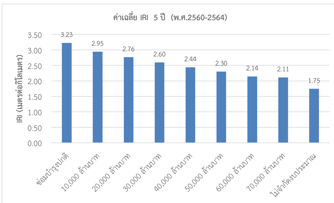
รูปที่ 4 กราฟแสดงค่า IRI เฉลี่ยในระยะเวลา 5 ปี ตามงบประมาณที่ได้รับในแต่ละปี
