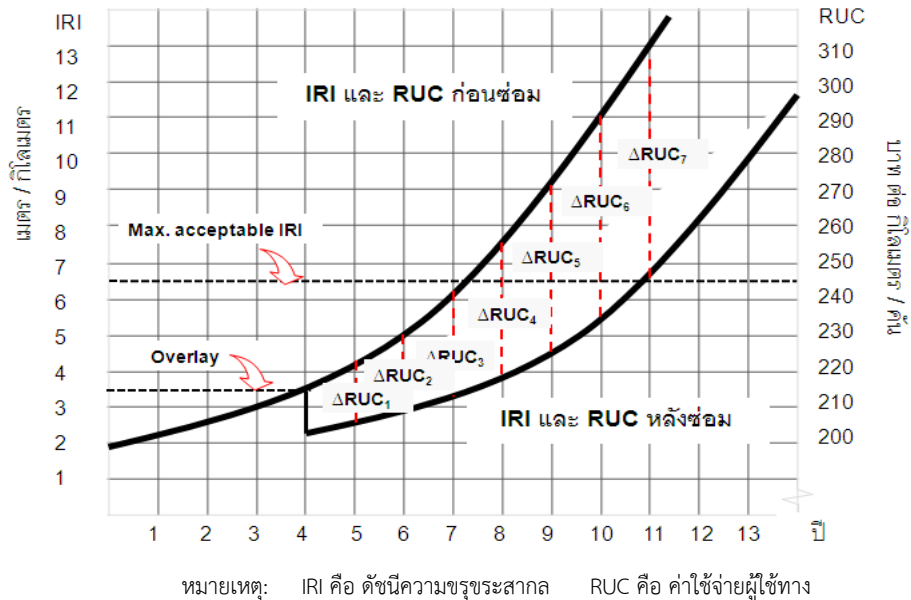
รูปที่ 1 การคำนวณผลประโยชน์ของผู้ใช้ทาง
