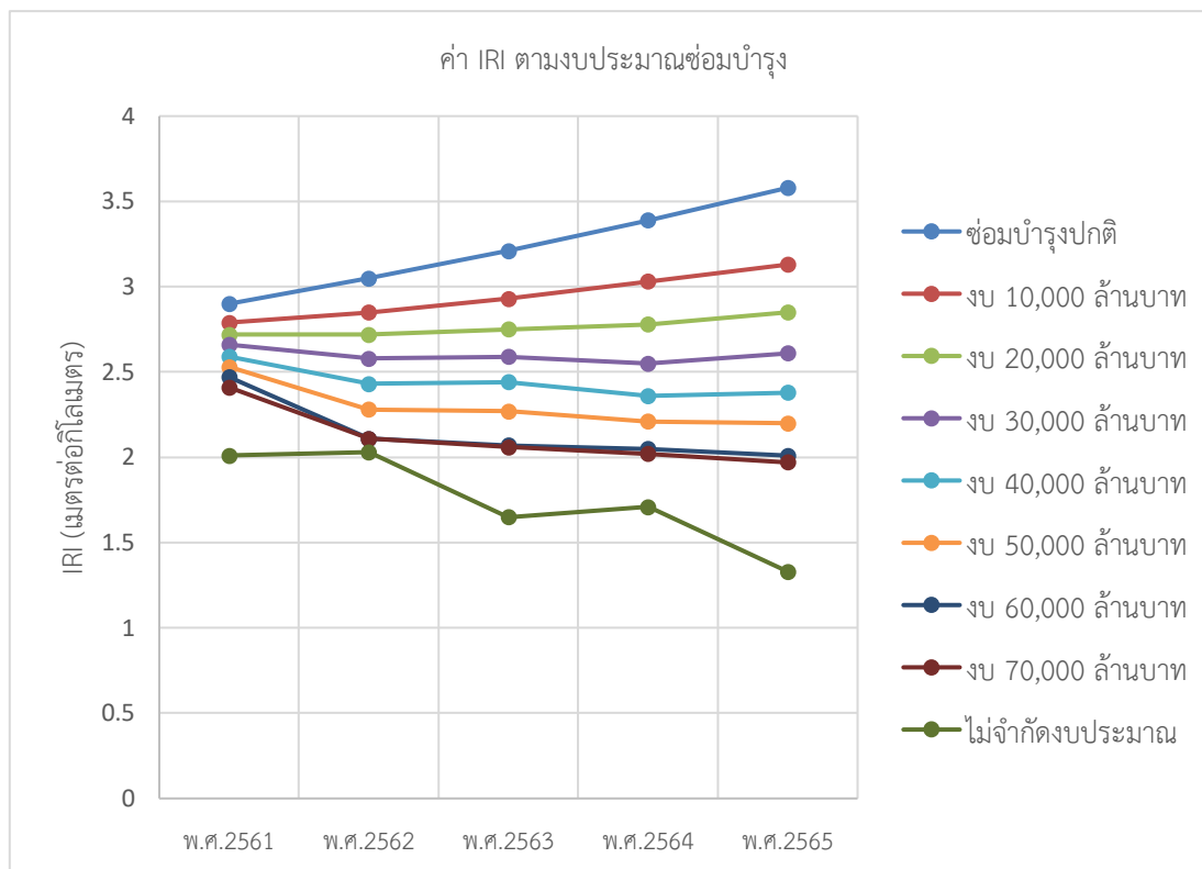
รูปที่ 3 กราฟแสดงค่า IRI ของแผนงบประมาณที่ได้รับในแต่ละปี
