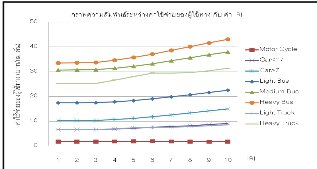
รูปที่ 3-6 กราฟแสดงความสัมพันธ์ระหว่างค่าใช้จ่ายของผู้ใช้ทางกับค่า IRI ต่างๆ
