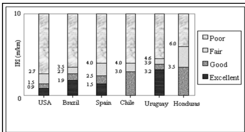
รูปที่ 3-18 การประเมินระดับการให้บริการของสายทางในประเทศต่างๆ โดยใช้ค่า IRI
