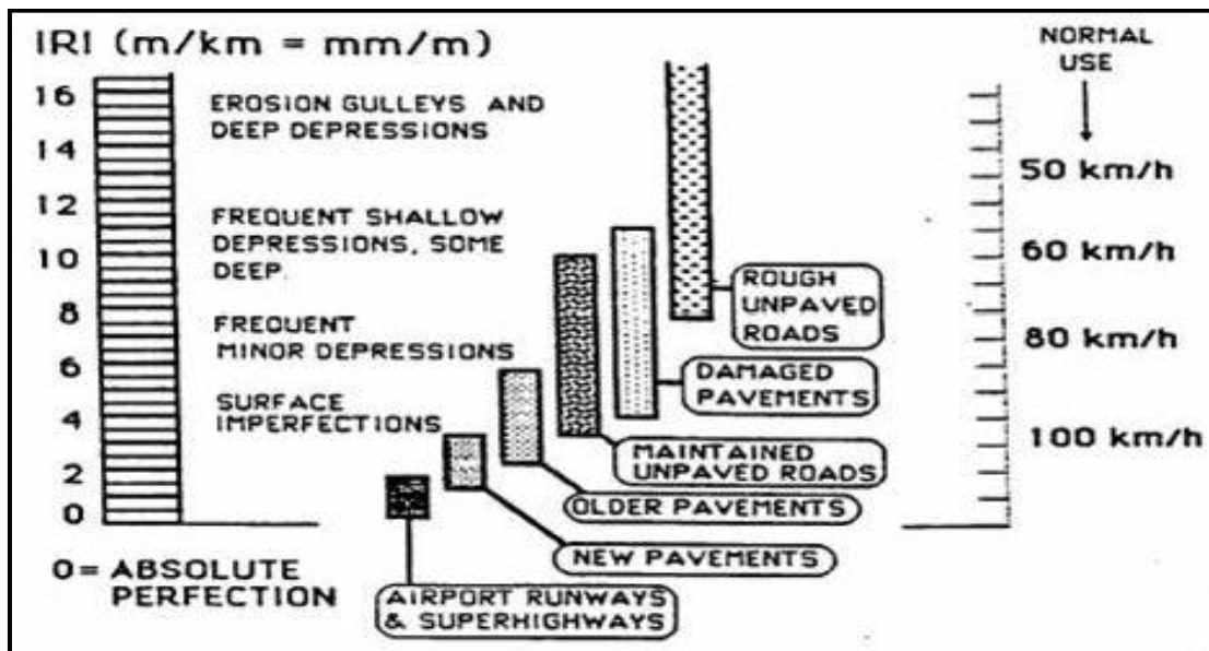
รูปที่ 3-17 กราฟแสดงความสัมพันธ์ระหว่างค่า IRI กับ ความเร็วยานพาหนะ (Paterson,1987)
