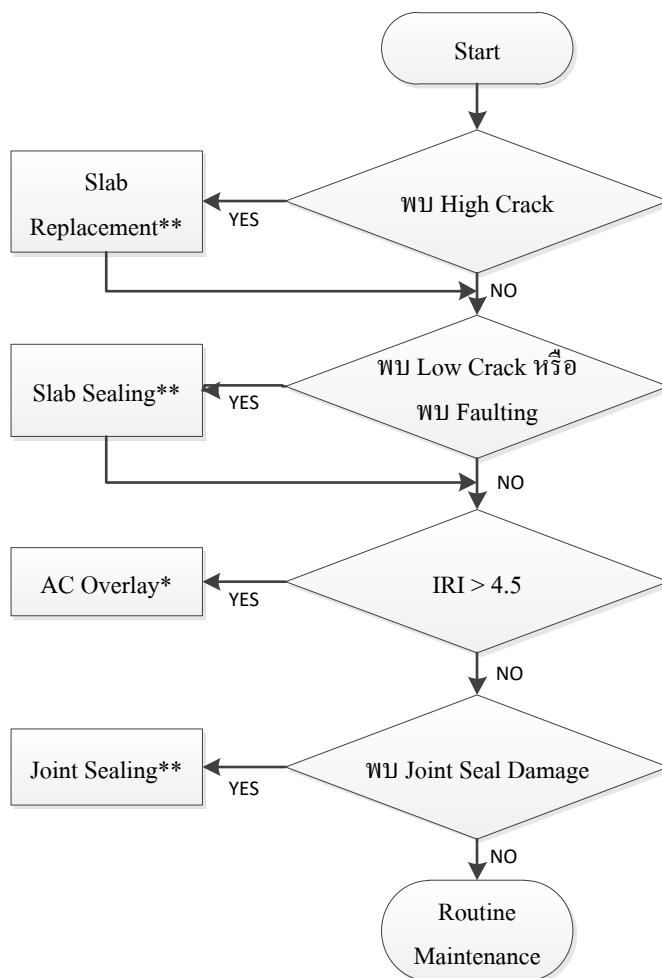
รูปที่ 3-16 ขั้นตอนการพิจารณาวิธีซ่อมบำรุงผิวทางคอนกรีต
