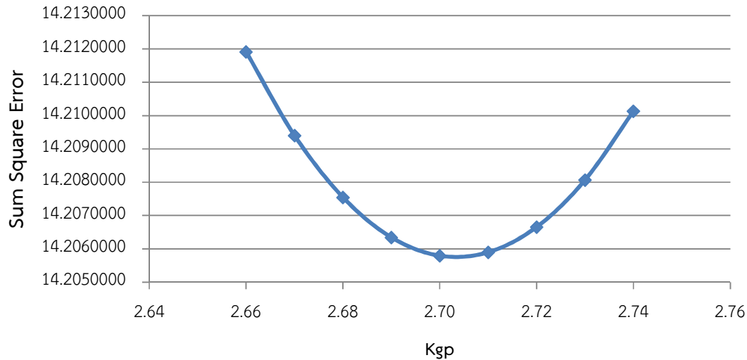
รูปที่ 2-5 ค่าผลรวมกำลังสองของความคลาดเคลื่อน เมื่อคำนวณโดยใช้ค่า Kgp ต่างๆ
