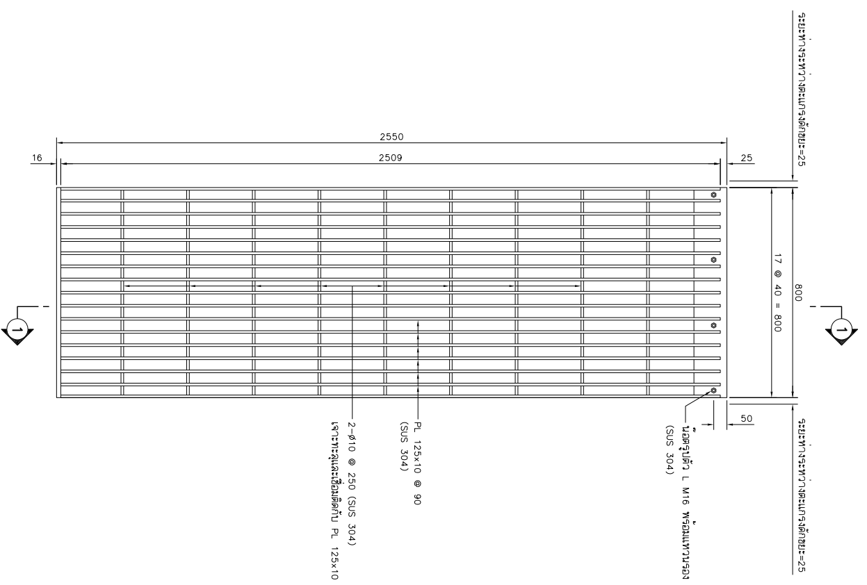
รูปด้านหน้าสะพานตะแกรงดักขยะ SUS 304 (จำนวน 3 ชุด) มาตราส่วน 1:10
