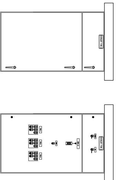
EXHAUST FAN PANEL 2
