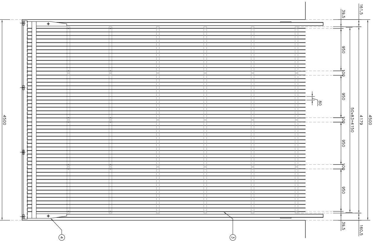
รูปด้านหน้า นทพ.ร.ว.น 1:25
