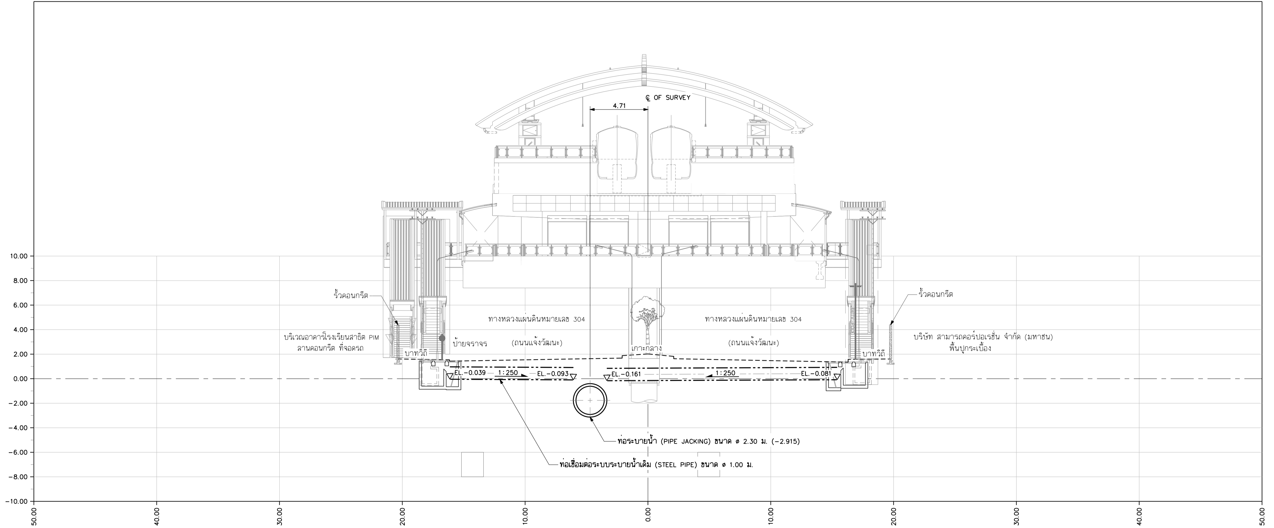
รูปตัดตามขวาง 13-13 กม. 7+949.239 มาตรฐาน 1:150
