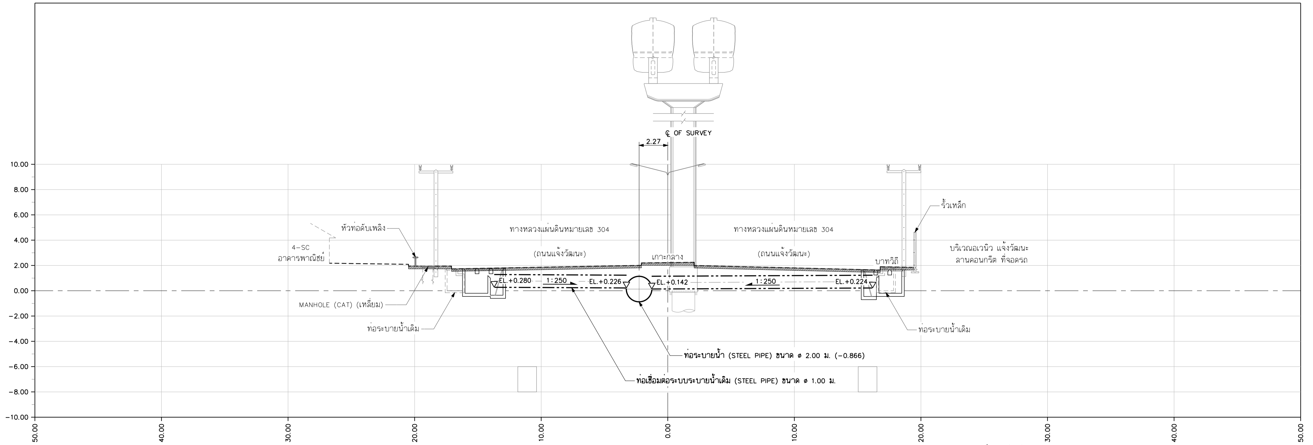
รูปตัดตามขวาง 8-8 กม. 4+570.520 มาตราส่วน 1:150
