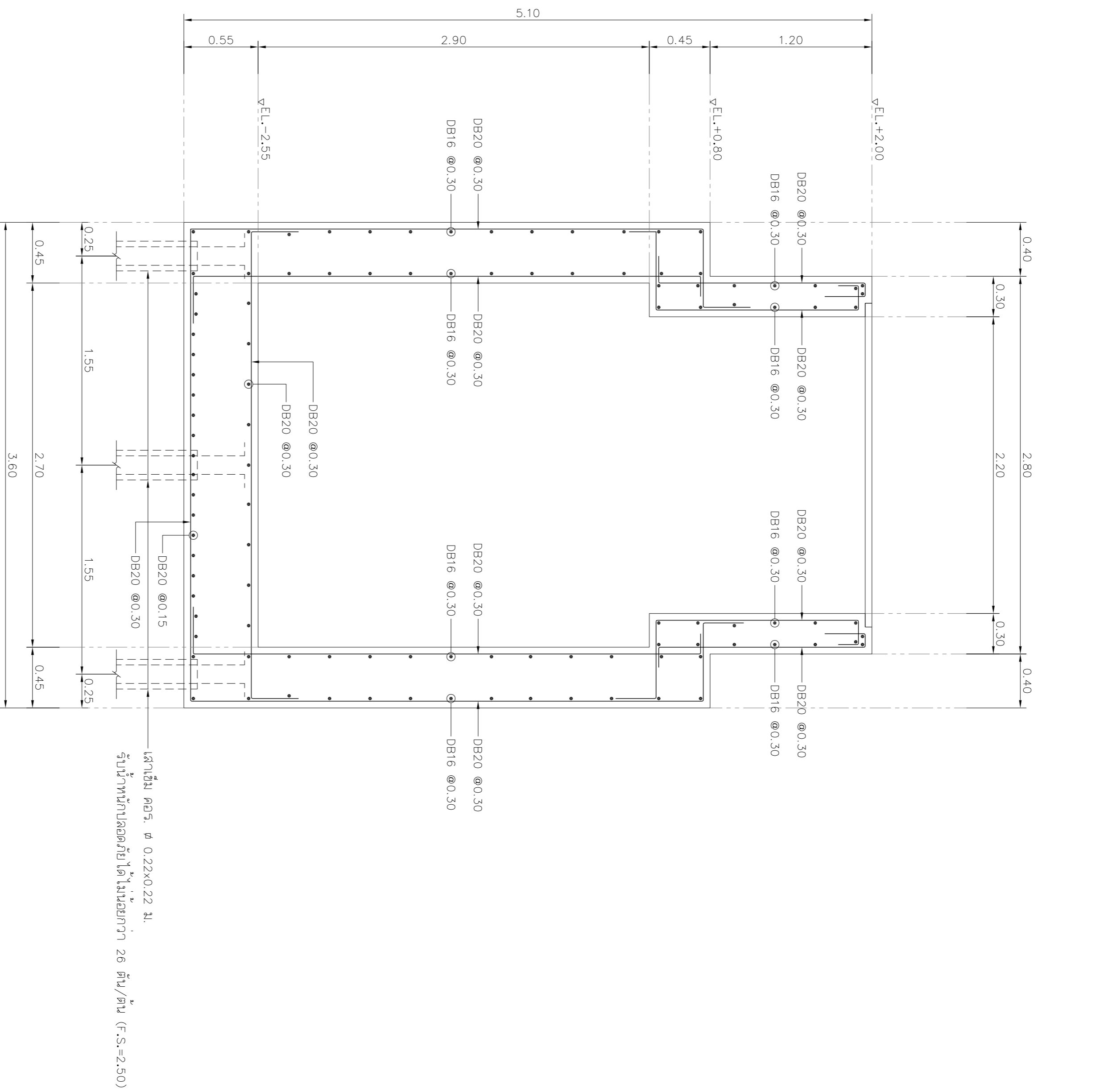
รูปตัด ค-ค มาตราส่วน 1:25
