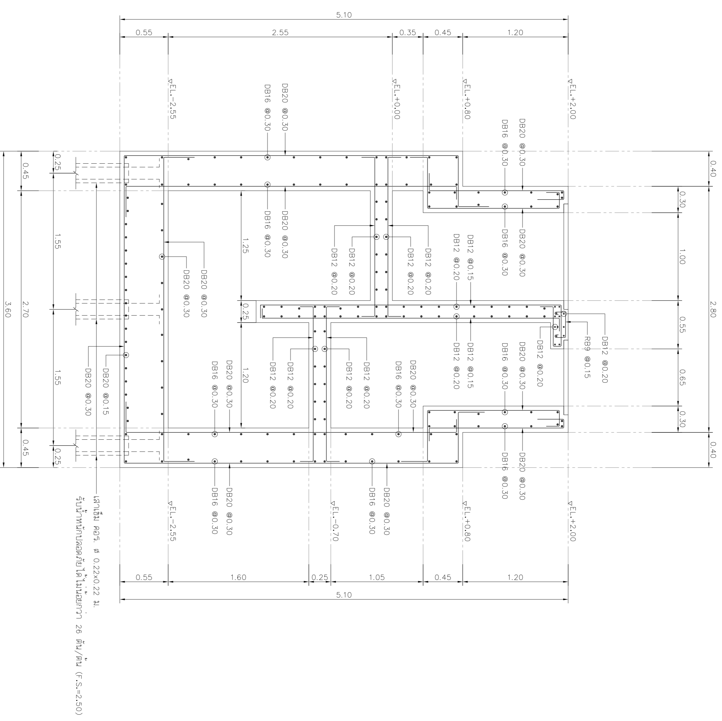
รูปตัด ง-ง มาตราส่วน 1:25
